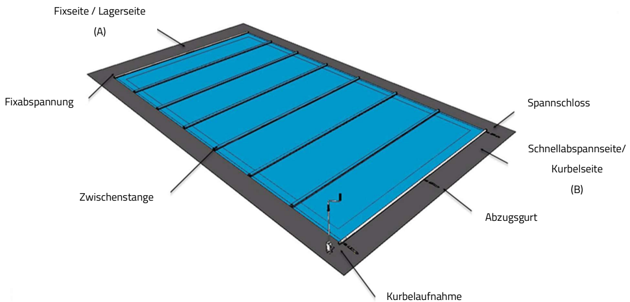
Abbildung 2-1: Aufbau
