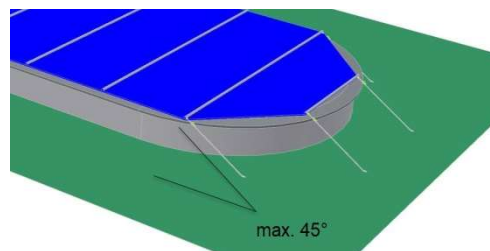
Abbildung 2-7: Erhöhter Beckenrand
